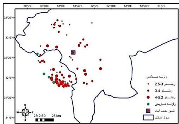
شکل ۶. زمین‌لرزه‌های تاریخی و دستگاهی (۱۹۶۲-۲۰۱۴) در شعاع صد کیلومتری شهر نجف‌آباد
